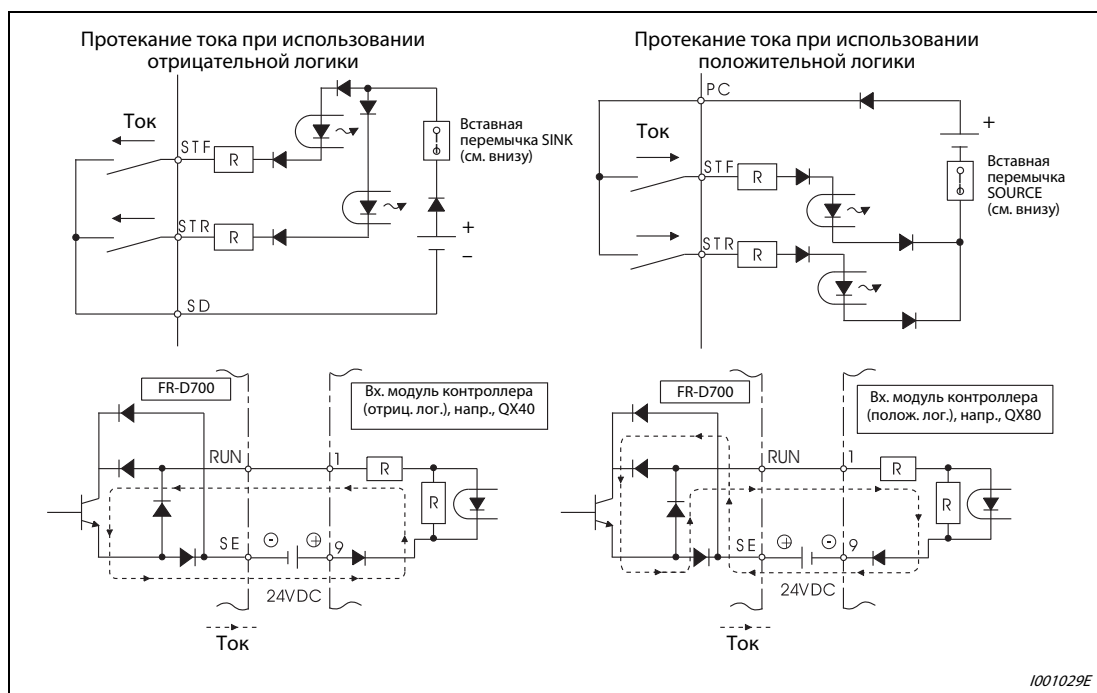
Рис. 3-15: Ток при отрицательной и положительной управляющей логике
