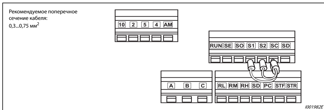
Рис. 3-6: Расположение клемм
