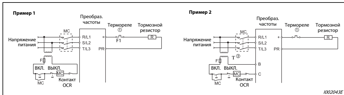
Рис. 3-25: Защитные схемы
