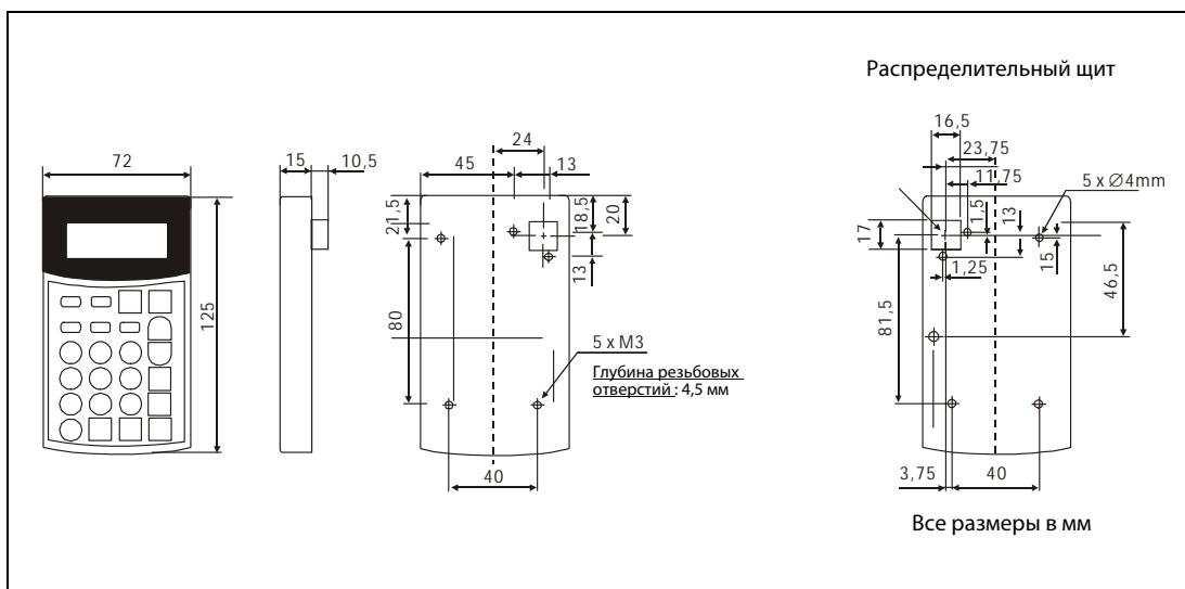
Рис. А-6: Пульт управления FR-PU04
