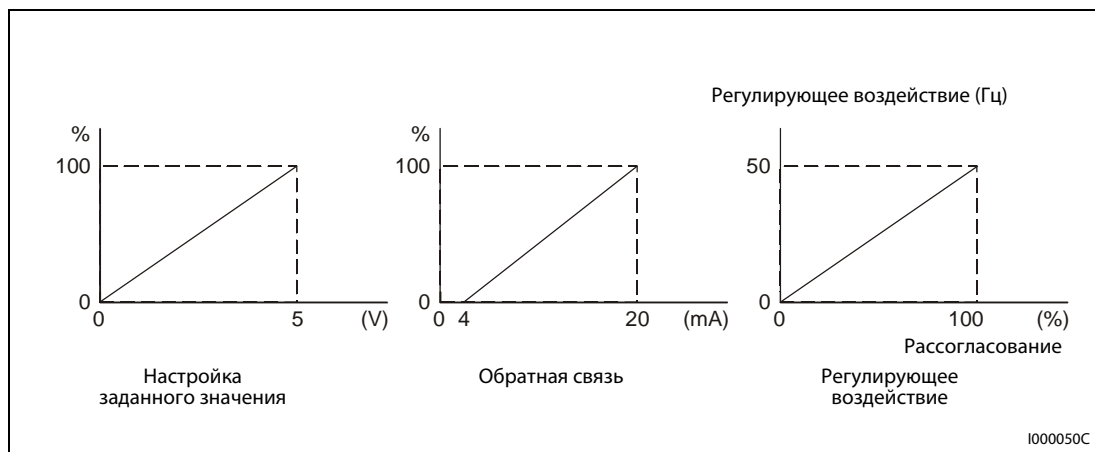
Рис. 6-129: Калибровка входов
