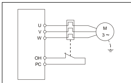
Рис. 6-36: Подключение внешней защиты двигателя
