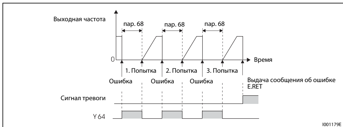
Рис. 6-76: Пример неудачных попыток перезапуска
