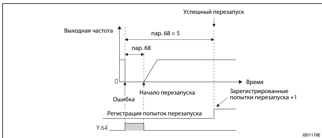
Рис. 6-75: Пример успешно выполненного перезапуска
