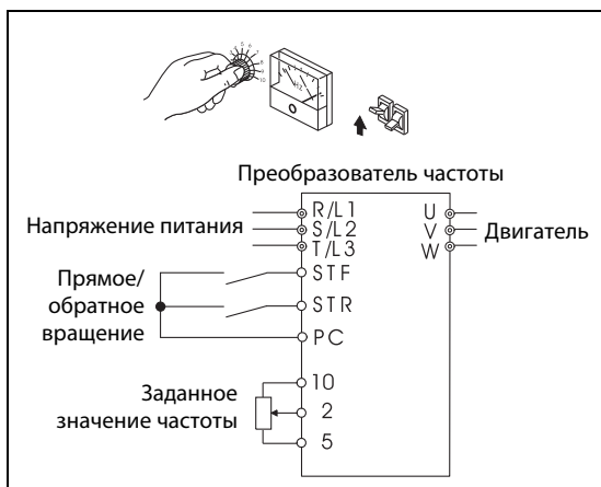
Рис. 6-91: Внешнее управление
