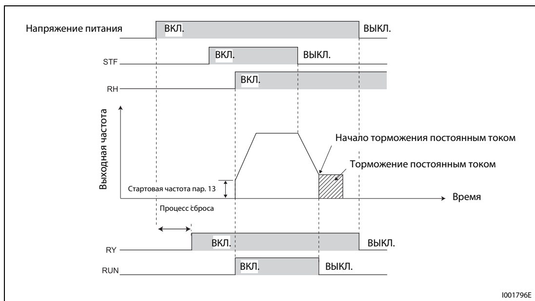
Рис. 6-51: Готовность к работе и работа двигателя
