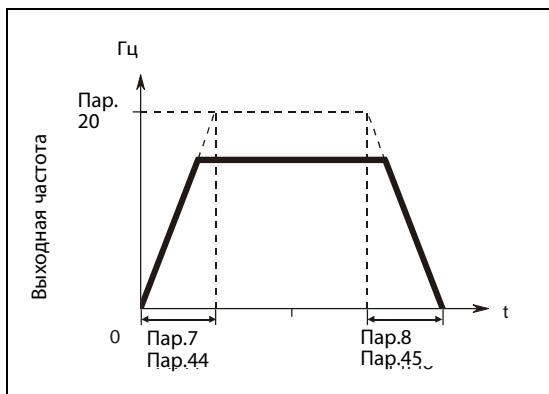
Рис. 6-27: Время разгона/торможения
