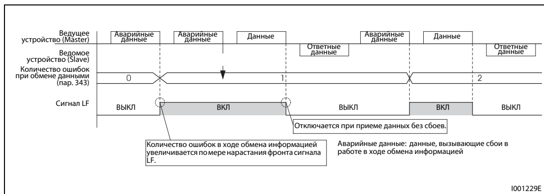
Рис. 6-117: Вывод сигнала LF
