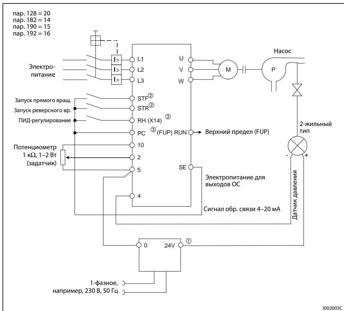
Рис. 6-124: Пример подключения при положительной логике
