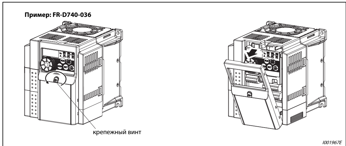
Рис. 2-1: Снятие передней панели
