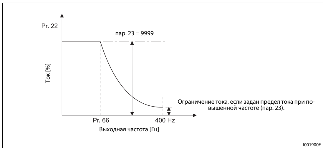
Рис. 6-6: Характеристика предельного тока
