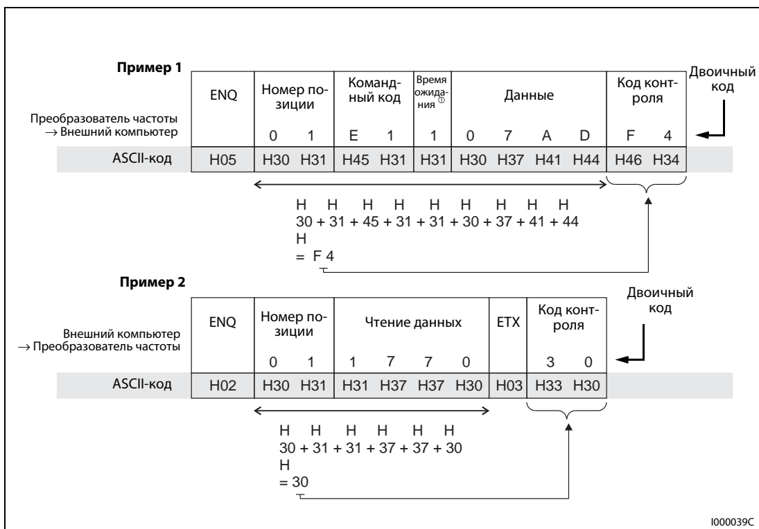
Рис. 6-110: Код контроля суммирования (примеры)
